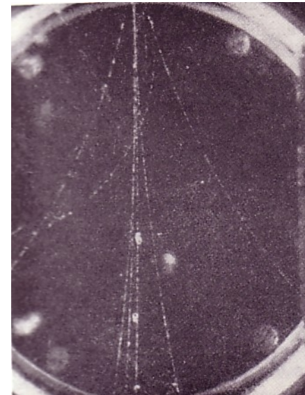
“Sciame” di raggio cosmico contenente alcune coppie e^+ e^-
